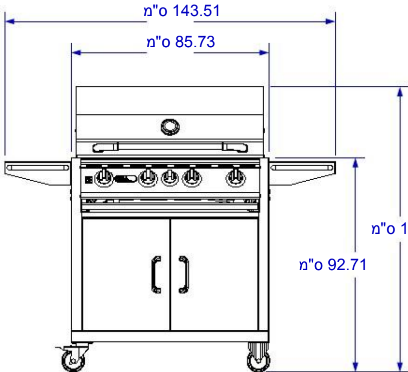
מבט חזיתי
